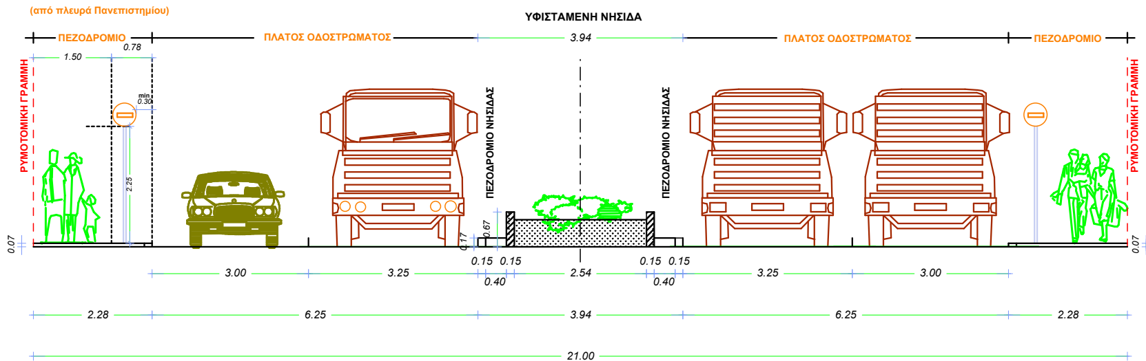
ΤΥΠΙΚΗ ΔΙΑΤΟΜΗ ΟΔΟΥ (ΚΛ. 1:100)
