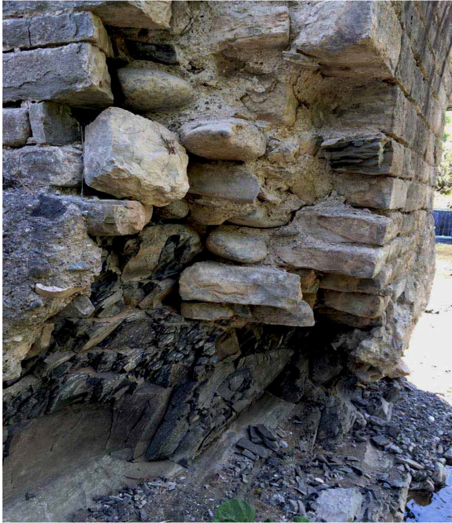
Γ.05.03. Αποκολλήσεις λίθων στο ανατολικό ακρόβαθρο
