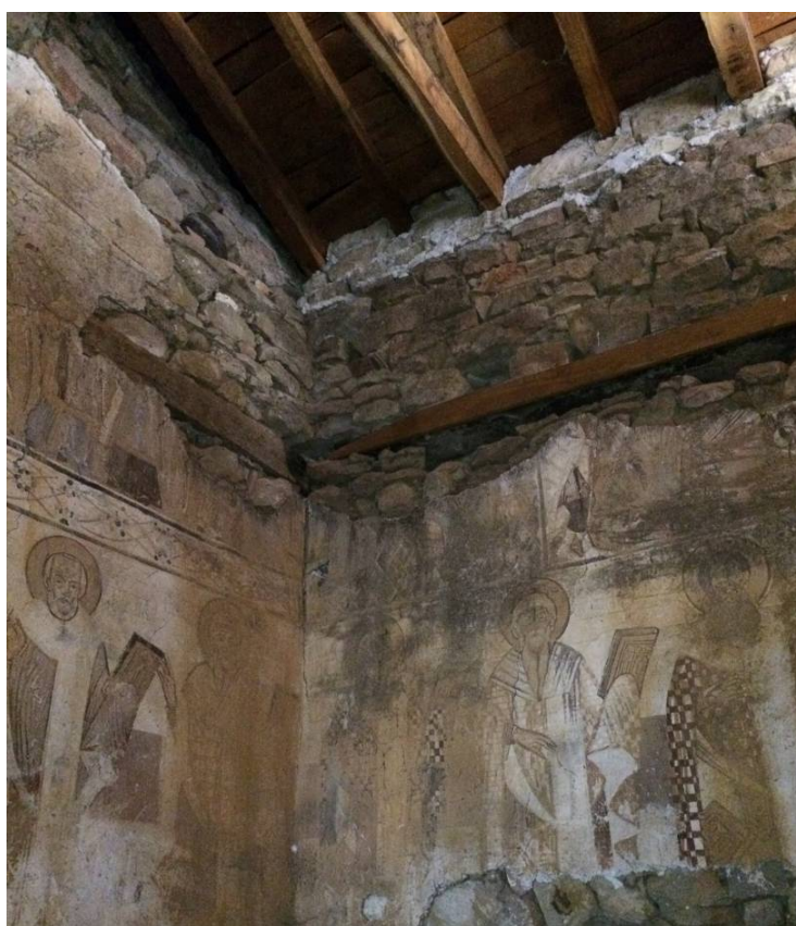
Ε.08.06. Ρηγμάτωση στη νοτιοδυτική γωνία
