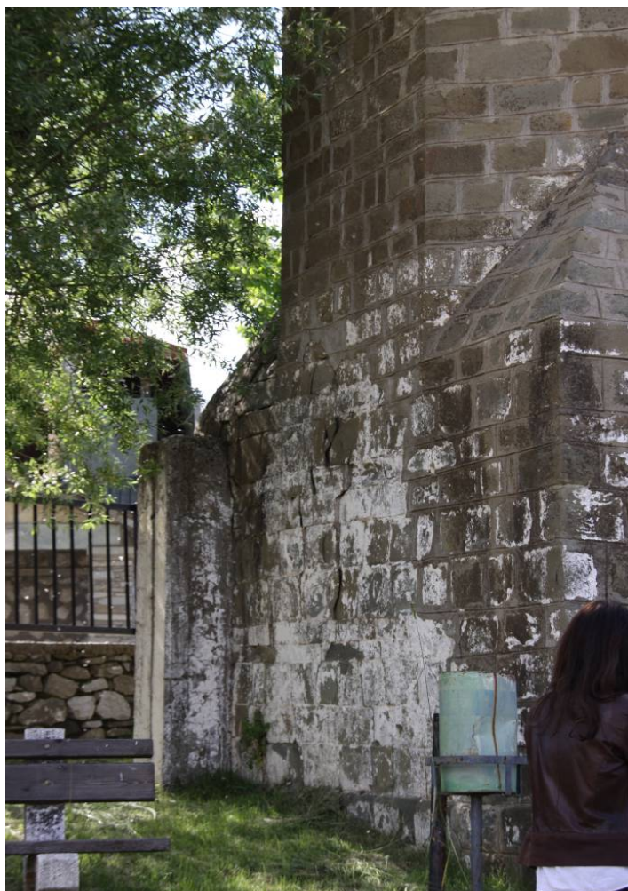
Ε.09.08. Ρωγμές στη βάση του κωδωνοστασίου
