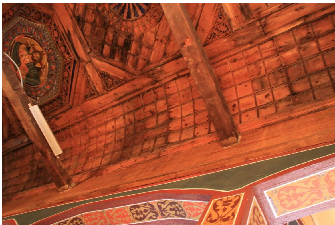
Ε.19.06. Εξόλκευση οριζόντιων ελκυστήρων και προσβολή τους από υγρασία
