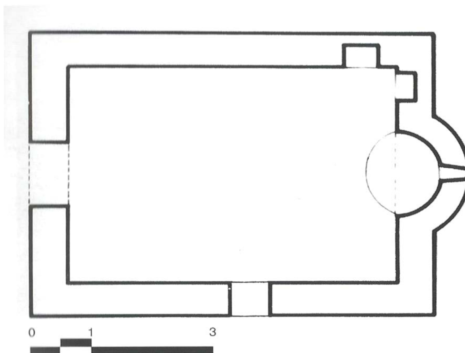
Ε.25.00. Παναγιά, Αγία Παρασκευή, Κάτοψη
