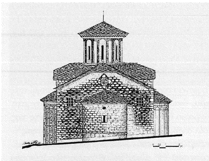
Ε.24.02. Παλιουριά, Μονή Ευαγγελίστριας, Καθολικό, Α. όψη
