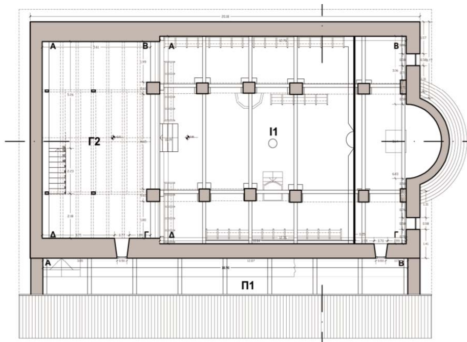
E.20.01 Κάτοψη ναού
