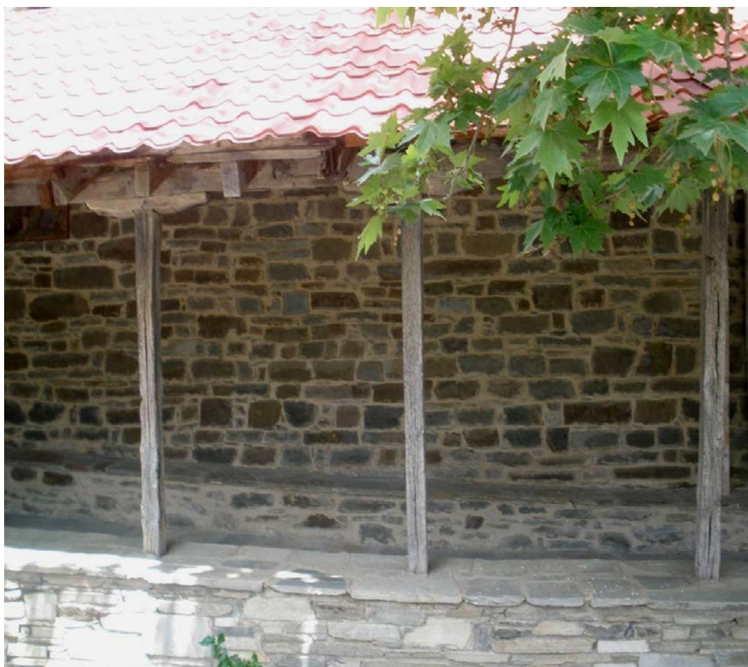
Ε.15.06. Σκελετός εξωνάρθηκα σε κατάσταση φθοράς
