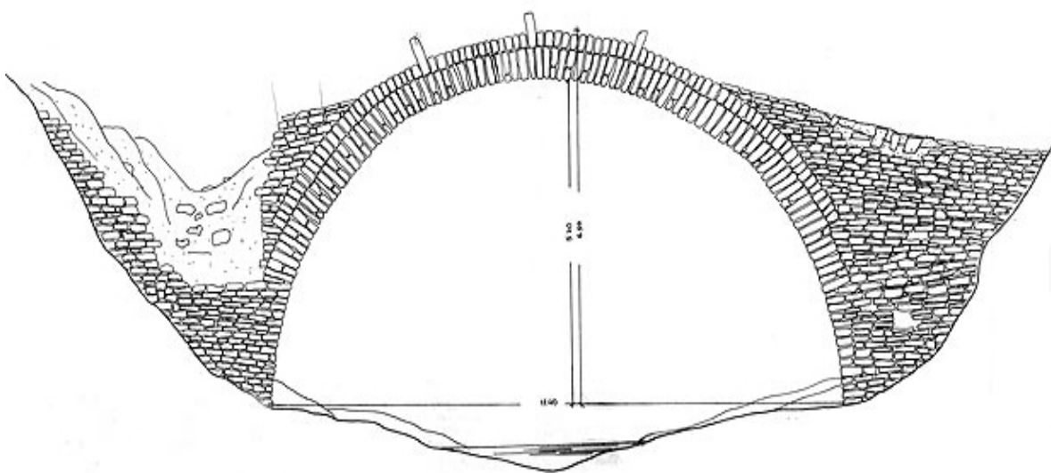
Γ.04.01. Βόρεια όψη. Αποτύπωση κατάστασης πριν την έναρξη εργασιών αποκατάστασης
