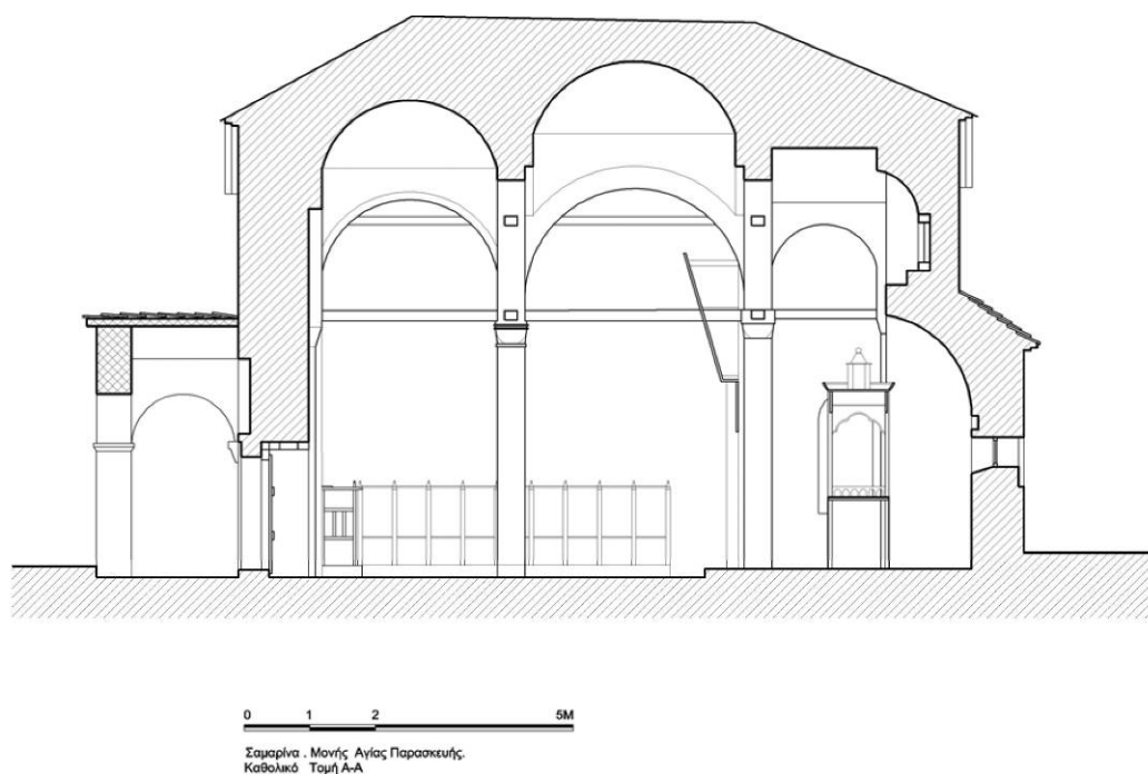
E.13.03. Τομή του Ι.Ν.
