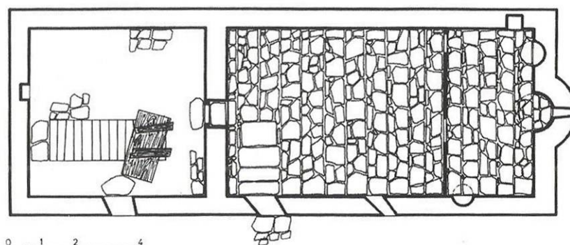
E.21.00. Κάτοψη ναού
