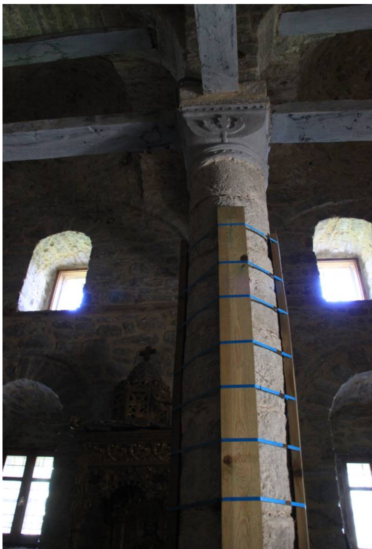
Ε.13.06. Πρόχειρη περίσφιξη υποστυλωμάτων
