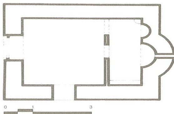
Ε.02.00. Πυλωροί, Άγιοι Απόστολοι, κάτοψη ναού
