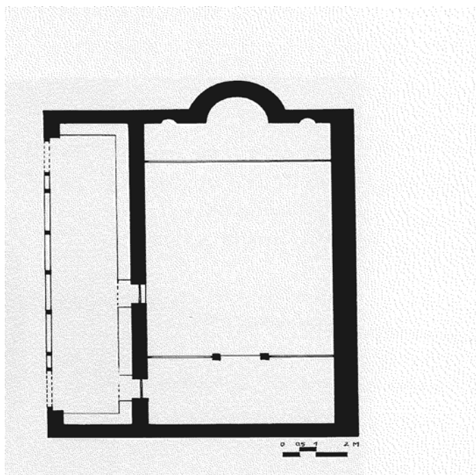
Ε.03.00. Κάτοψη ναού
