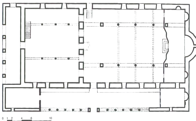
Ε.09.01. Σαμαρίνα, Μεγάλη Παναγιά, κάτοψη
