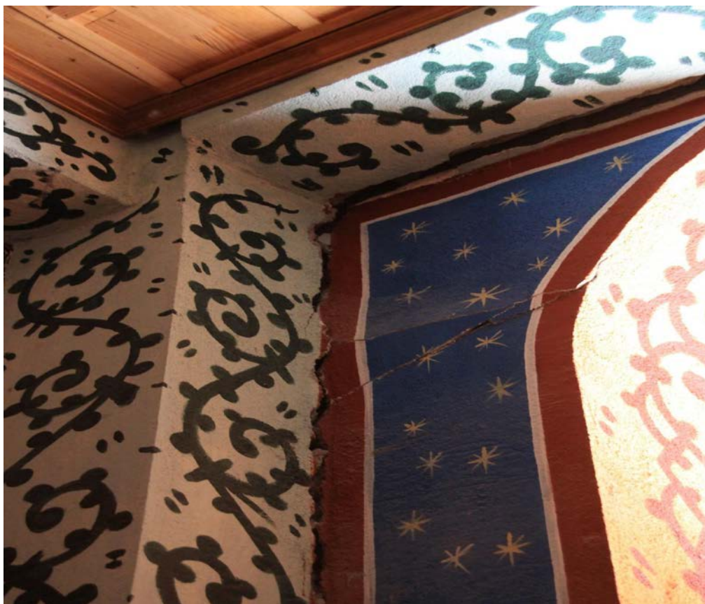
Ε.19.07. Διαμπερείς οριζόντιες και κατακόρυφες ρωγμές σε θέση συναρμογής νεώτερου πλαισίου ο/σ με περιμετρικό τοίχο
