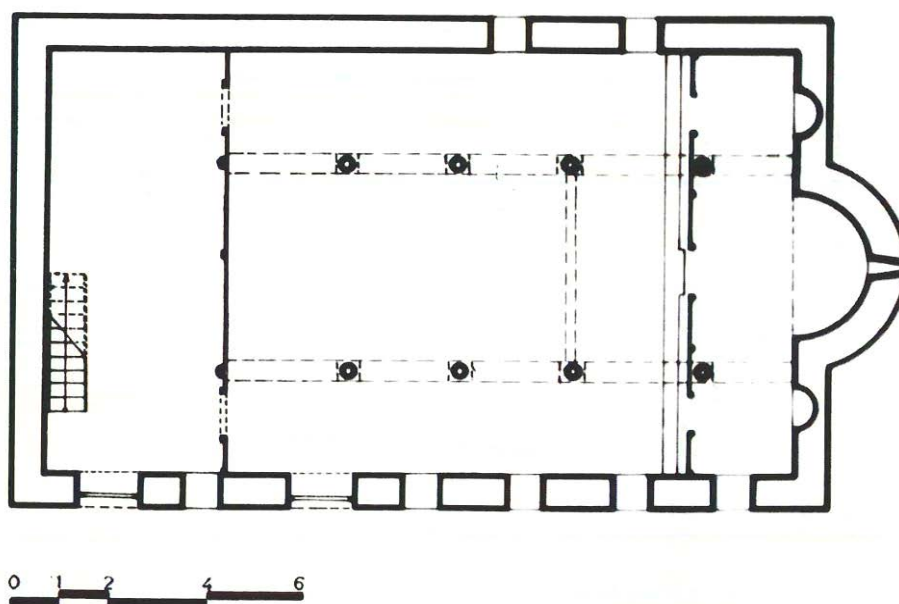
Ε.19.00. Σμίξη, Άγιος Νικόλαος, κάτοψη (αποτύπωση 1961)
