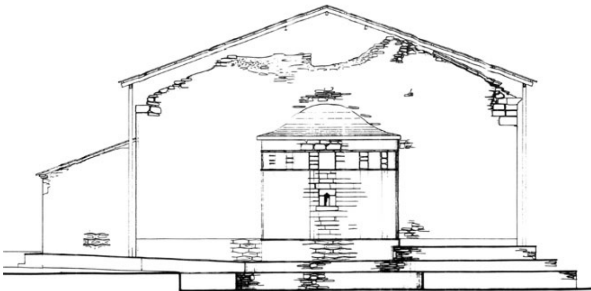
Ε.05.02. Ανατολική όψη ναού (Αποτύπωση βλαβών από το σεισμό του 1995)
