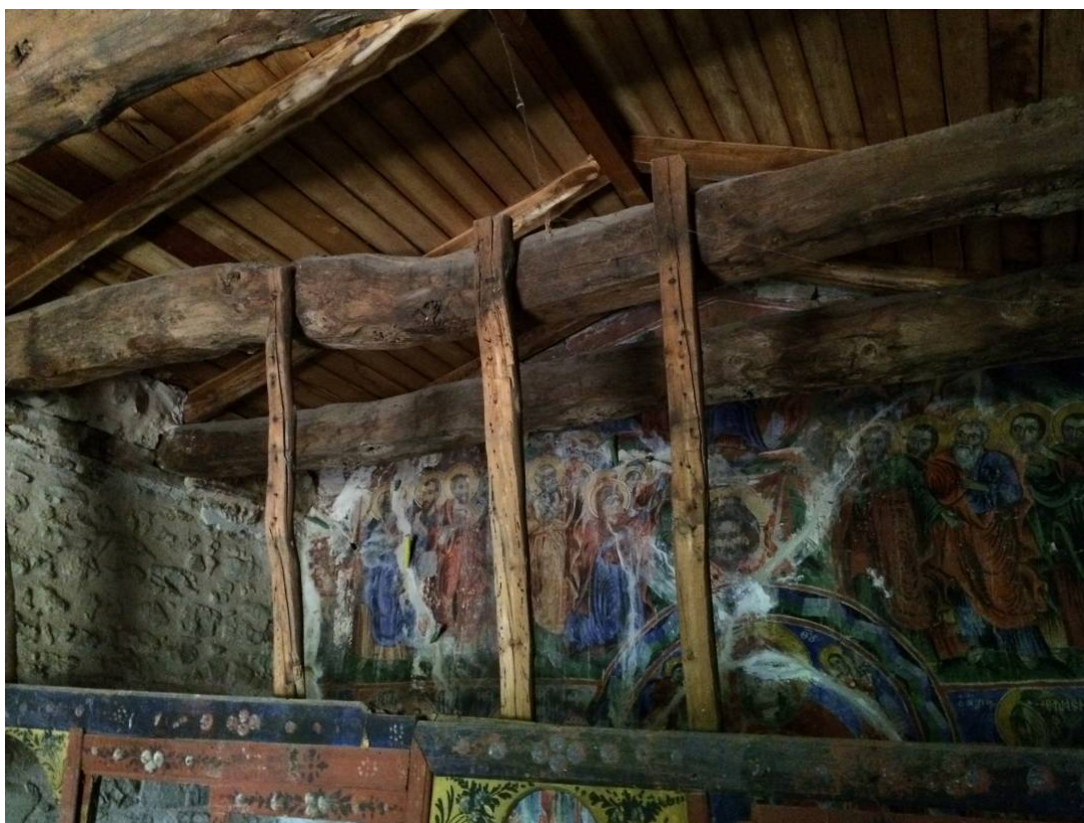
Ε.04.01. Ελκυστήρες στέγης
