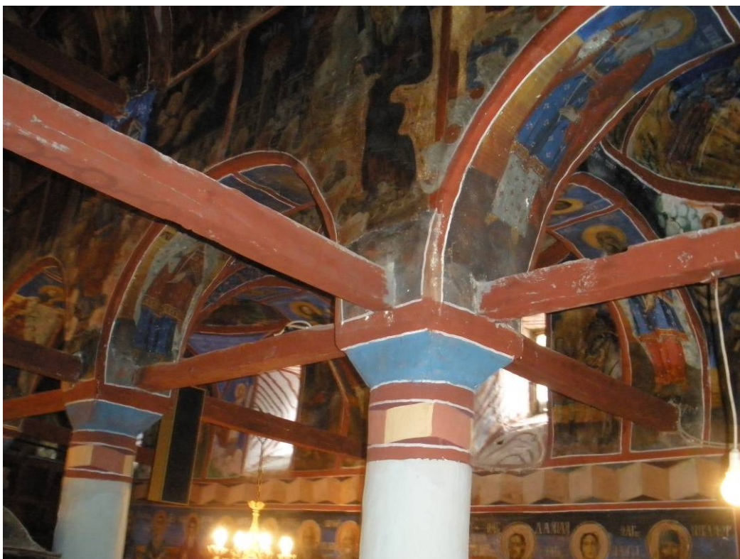
Ε.15.02. Εξολκεύσεις ξύλινων ελκυστήρων
