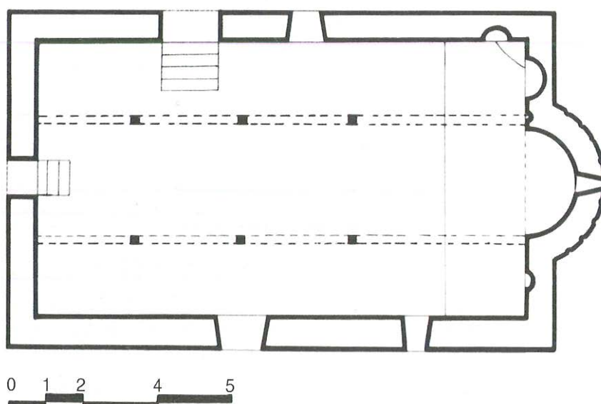
Ε.17.00. Σμίξη, Άγιος Αθανάσιος, κάτοψη
