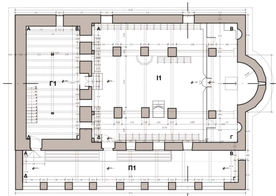
E.20.00. Κάτοψη ναού
