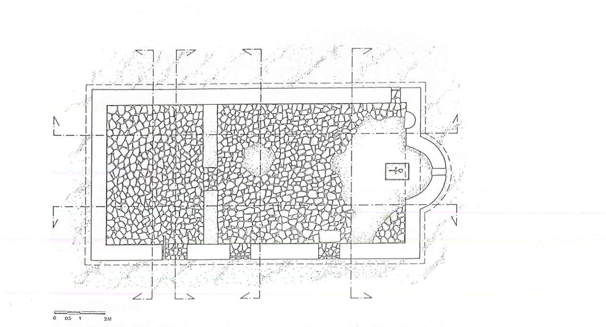
Ε.08.00 Κολοκυθάκι, Κοίμηση Θεοτόκου, κάτοψη
