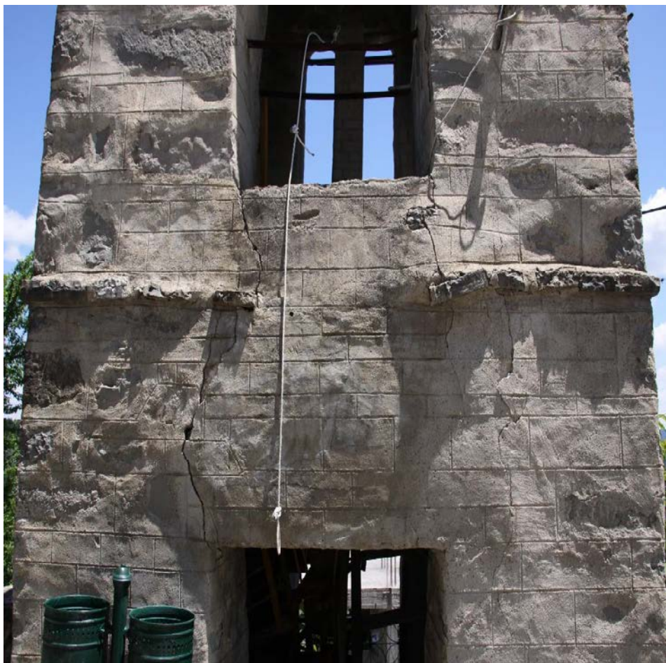
Ε.19.10. Βλάβες στο κωδωνοστάσιο
