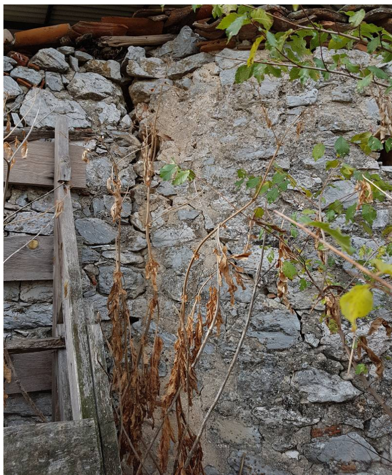
Ε.25.03. Έντονες ρηγματώσεις
