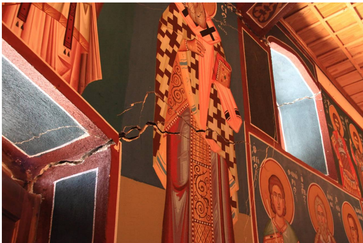
Ε.19.05. Ρωγμές μεγάλου εύρους στο νότιο τοίχο
