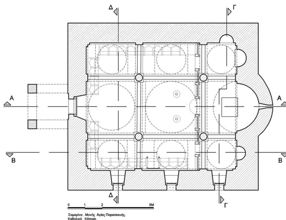
Ε.13.02, Κάτοψη του Ι.Ν.
