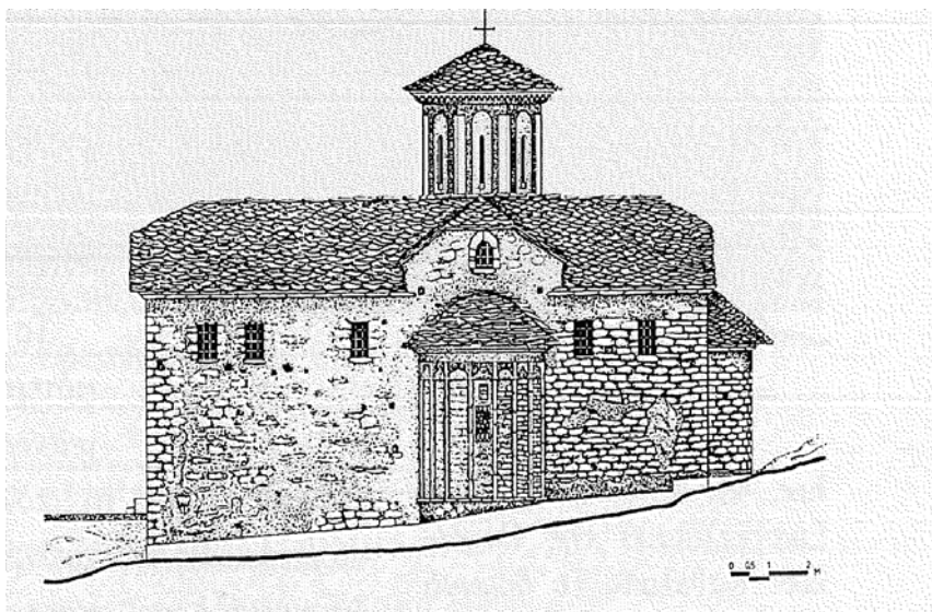
Ε.24.03. Παλιουριά, Μονή Ευαγγελίστριας, Καθολικό, Ν. όψη
