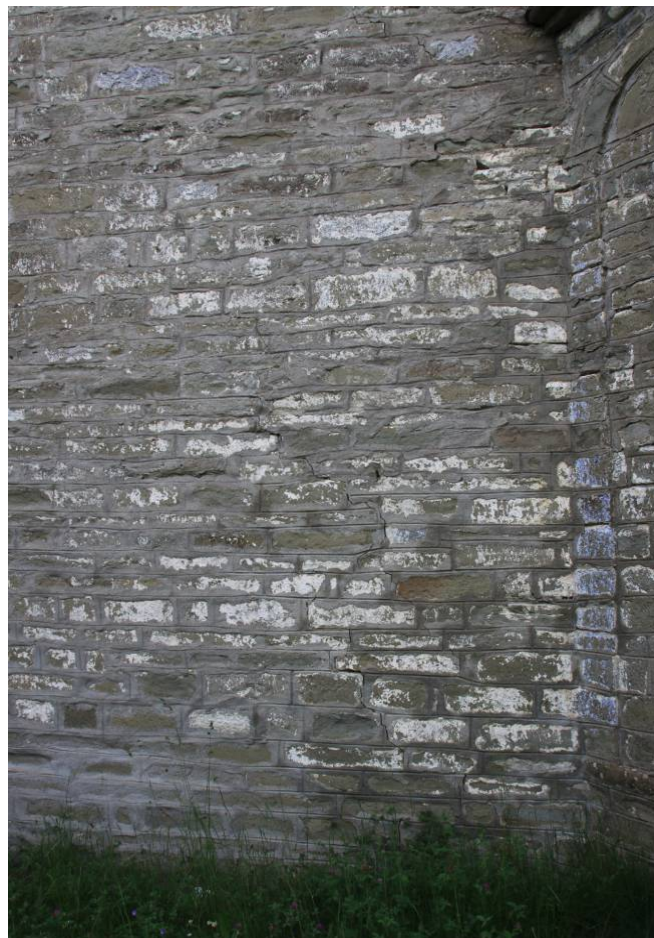
Ε.10.04. Ρηγματώσεις στον ανατολικό τοίχο
