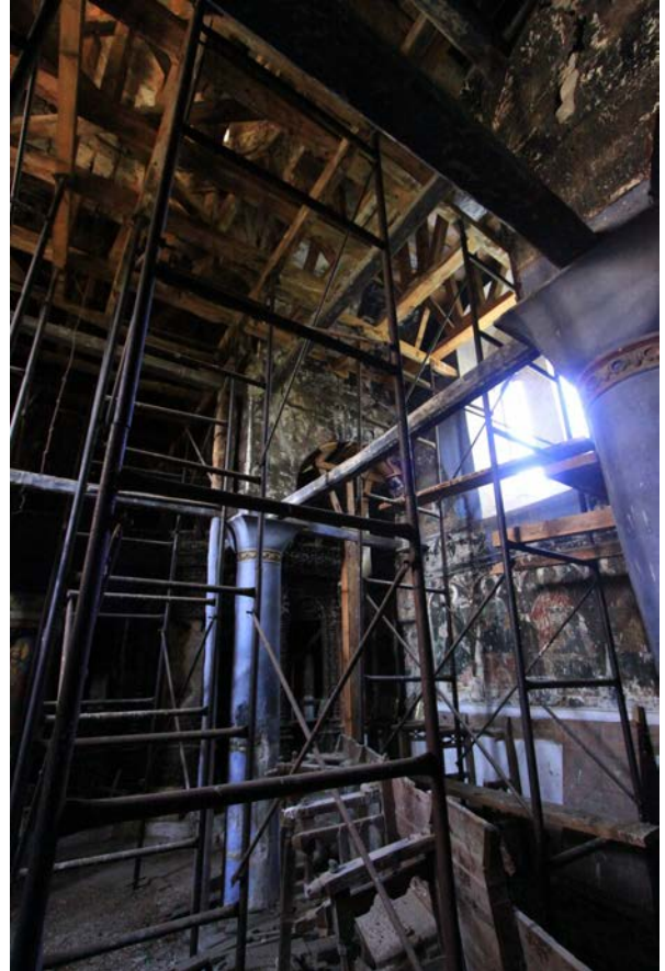
Ε.31.06. Εκτενής χρήση κριωμάτων
