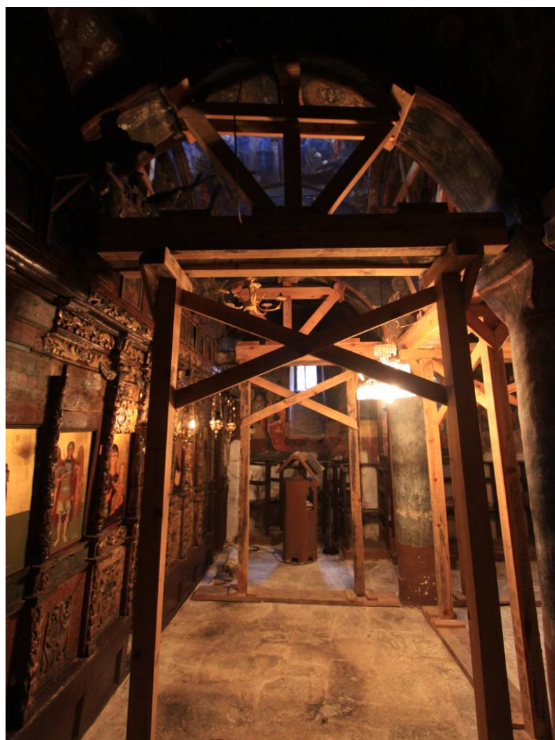
Ε.01.06. Κατακόρυφη υποστήλωση
