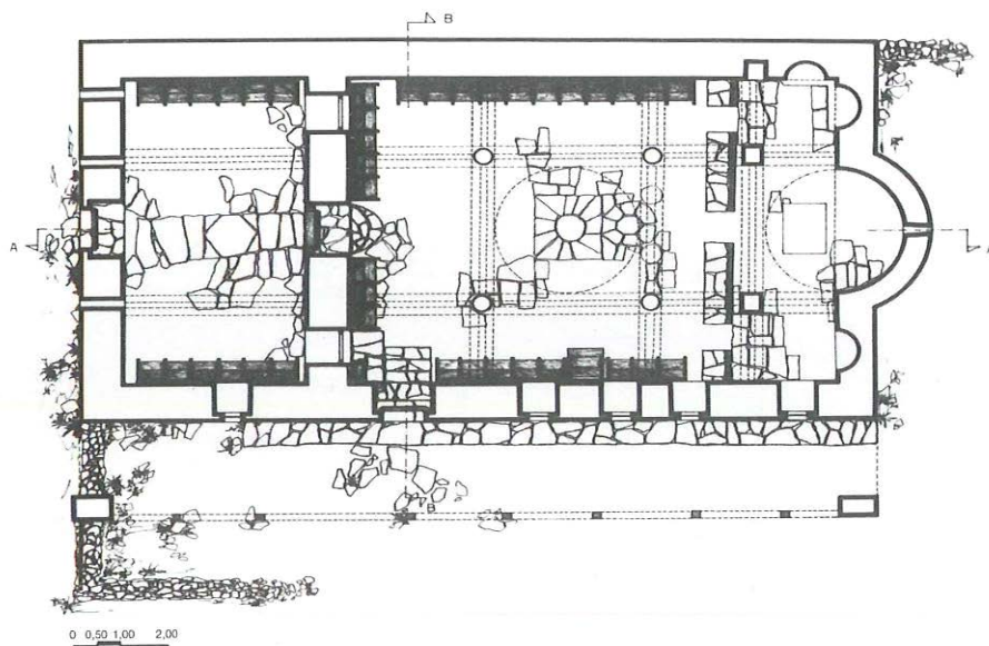
Ε.14.00. Σαμαρίνα, Μεταμόρφωση του Σωτήρος, κάτοψη
