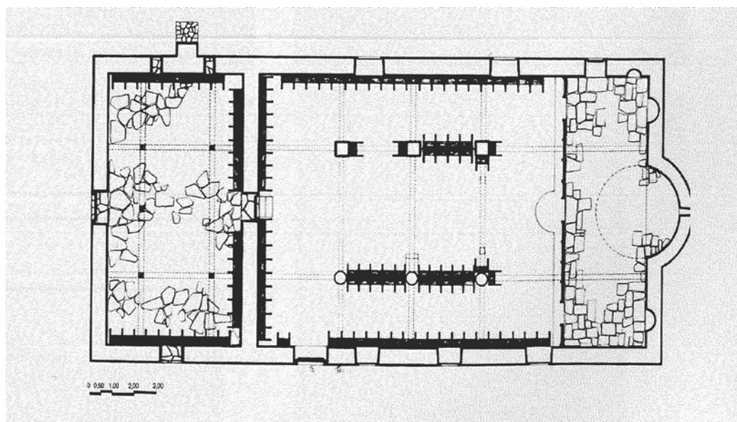
Ε.10.00. Σαμαρίνα, Μικρή Παναγιά, κάτοψη (αποτύπωση 1961)
