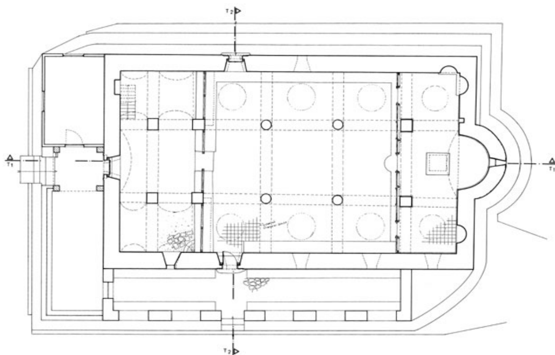
E.05.01. Κάτοψη του ναού
